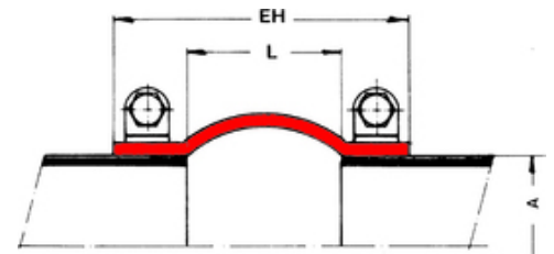
| Tip 12 - Compensator panza | dimensionare
