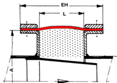
| Tip 21 - Compensator panza | dimensionare
