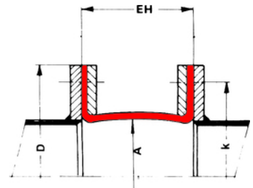
| Tip 31 - Compensator panza | dimensionare
