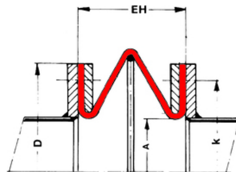
| Tip 33 - Compensator panza | dimensionare
