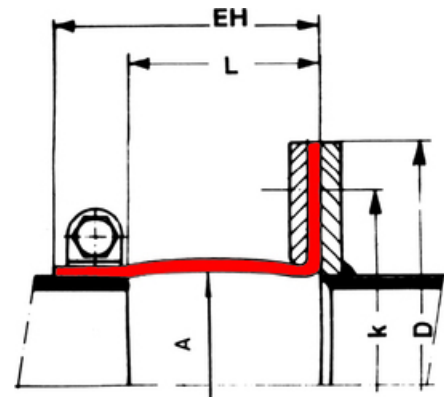
| Tip 51 - Compensator panza | dimensionare
