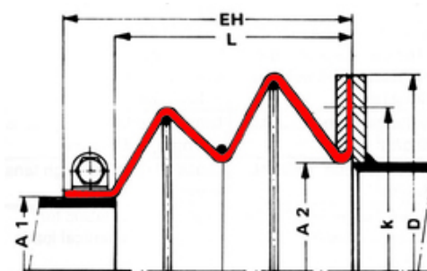
| Tip 54 - Compensator panza | dimensionare
